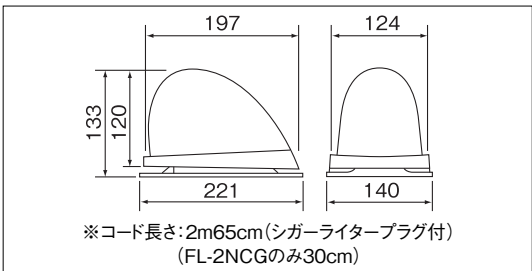
ゴムマグネット
