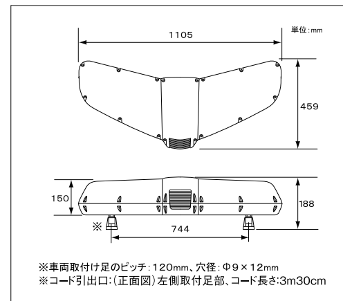
寸法図
