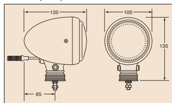
※取付用穴径φ10.5~φ11mm
