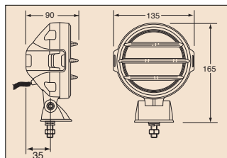
※取付用穴径φ10.5~φ11mm
